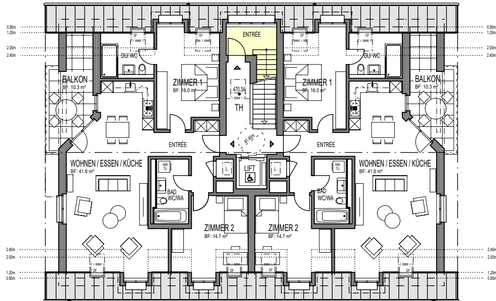
3½ Zi - DACHWOHNUNG WOHNUNG 15.6 WF: ca. 99.0 m 2
