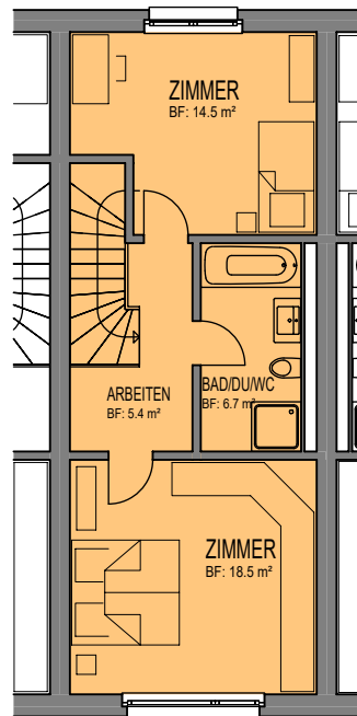
2. Obergeschoss
