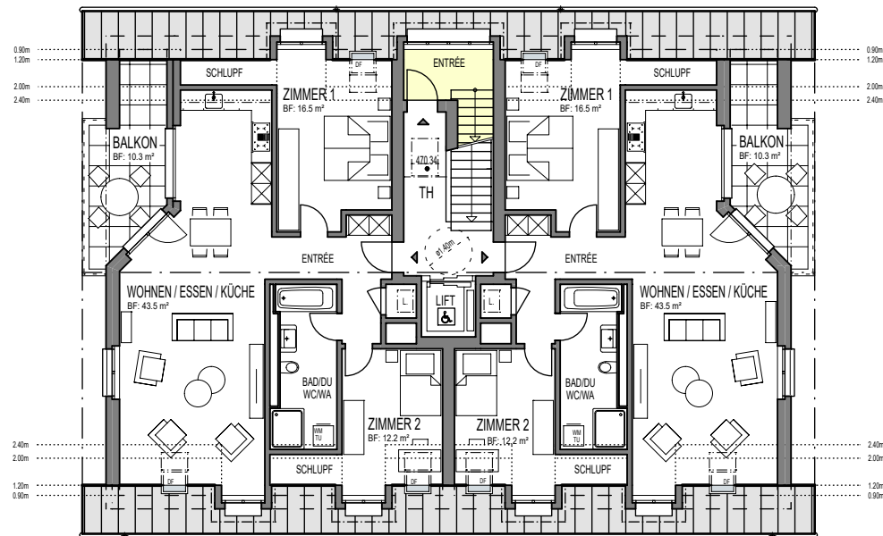
3½ Zi - DACHWOHNUNG WOHNUNG 15.6 WF: ca. 93.0 m 2
